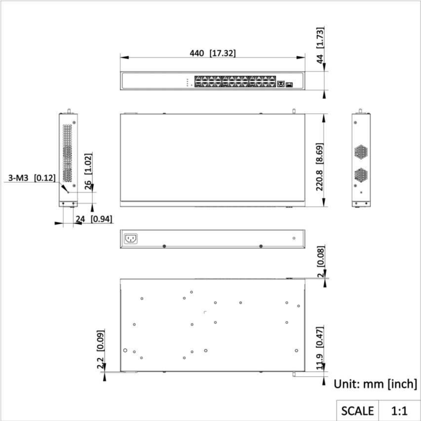
מידות - דגמי 24 פורטים (DS-3E1526P-EI / /M)
